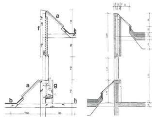
14.14. ábra. Szerkezeti részletek. a) Eredeti; b) új.
