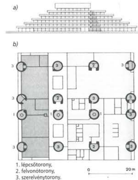
17.24. ábra. F. W. Kraemer: BP irodaépület, Hamburg, 1965.
