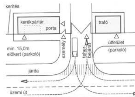
1.27. ábra. Bejárat (teher- és személybejárat) kialakítása.
