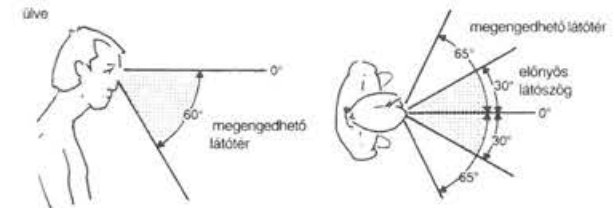
3.39. ábra. Függőleges látótér. 3.40. ábra. Vízintes látótér.
