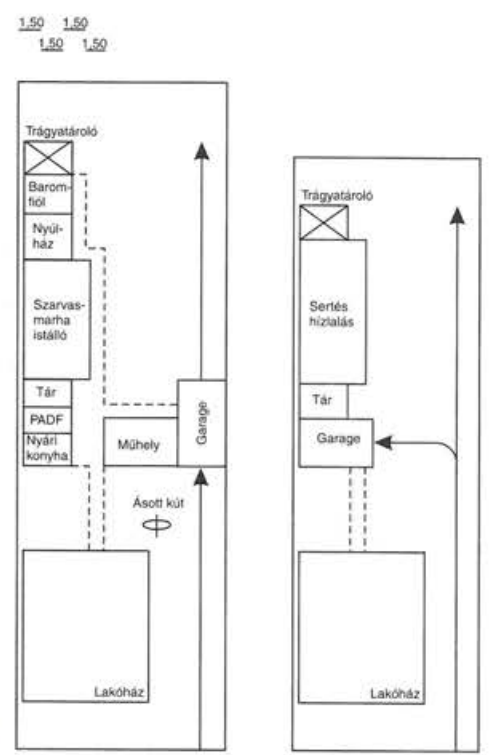
2.1. ábra. Oldalhatáron álló beépítés.
