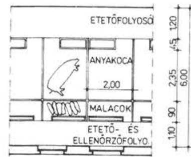
2.23. ábra. Egysoros fiaztatóól malacrekessel.
