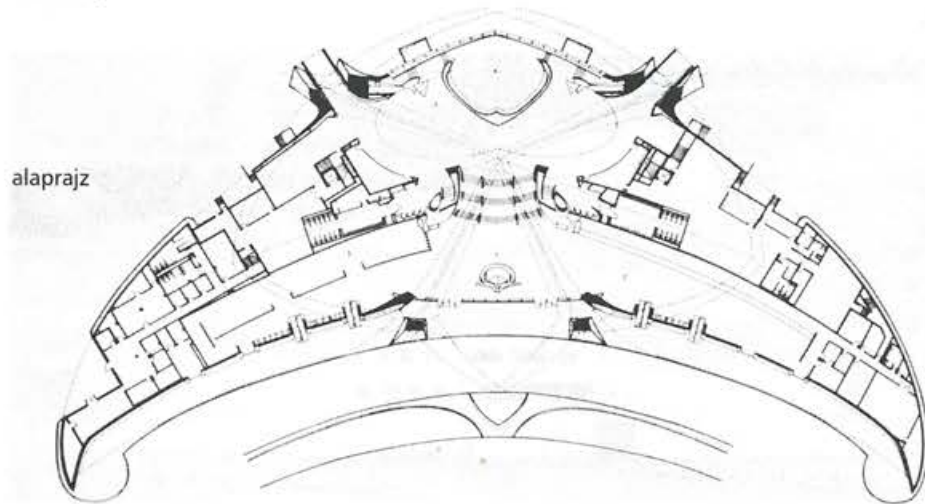
5.23. ábra. TWA utasforgalmi csarnok, New York (E. Saarinen, 1956–1962).
