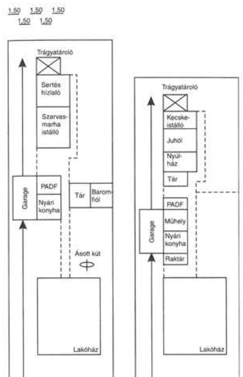
2.2. ábra. Szabadon álló beépítés.
