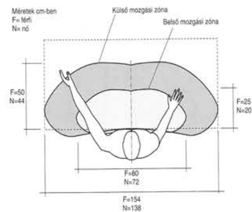
3.21. ábra. Kézrel elérhető munkaterület zónái.
