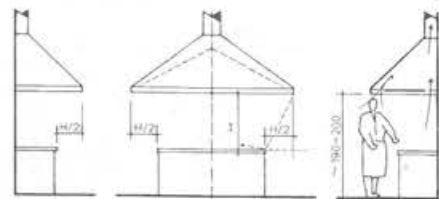
6.31. ábra. Elnívók helyigénye. H = asztal és elszívó közötti magasság.
