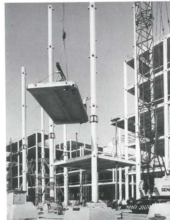
18.49. ábra. A Haditengerészet javítóüzeme – Garden Island/Sydney/Ausztrália, 1985 (Harry Seidler & Ass.). A nagy fesztávolságú, nagy teherbírású, többszintes, daruzott műhelyépület egyedi előregyártású, utófeszített vasbetonszerkezettel készült.
