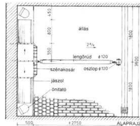
2.29. ábra. Állásos lóistálló alaprajzi részlete és metszete.
