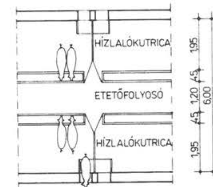
2.21. ábra. Kétsoros hízódisznóú kikutóval.
