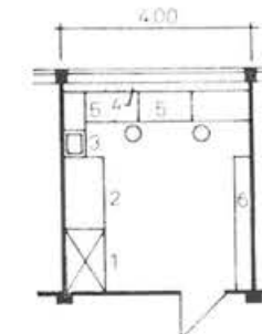
6.51. ábra. Frankfurt/M. Botanikai Intézet laboratóriuma.
