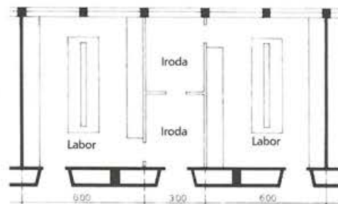
6.42. ábra. Egyforma laboregységek csoportosítása.
