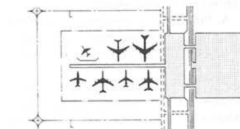
U-alakú elrendezés
