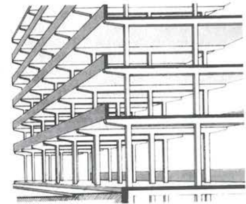
17.8. ábra. Betonszerkezet konzolokkal (H. Schmitt nyomán).
