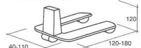
1.57. ábra. Kézi targoncák méretei.
