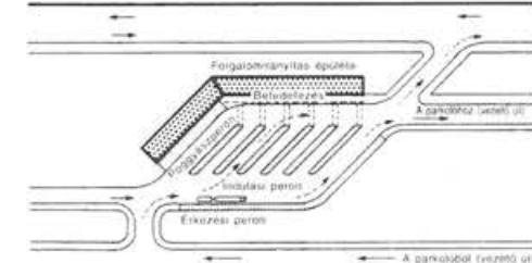
5.13. ábra. Autóbusz-pályaudvarok, forgalmi sémák.
