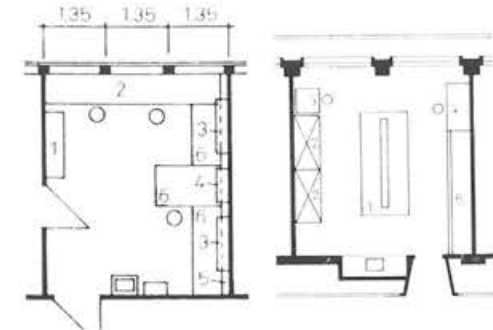
6.49. ábra. Tübingen, biológiai laboratórium.
