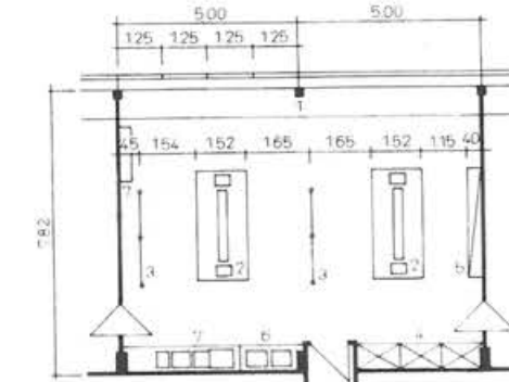
6.35. ábra. Hamburg, Deutsche Erdöl AG kutatólaboratórium.
