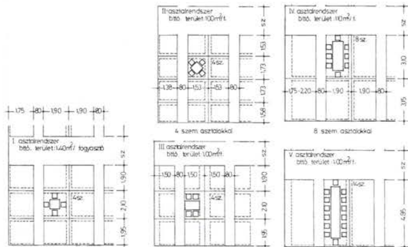
7.25. ábra. Asztalok elhelyezési változatai.
