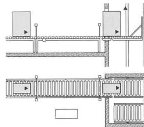
1.62. ábra. Görgősor.
