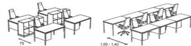
3.43. ábra. Közlekedők íróasztalok körül.
