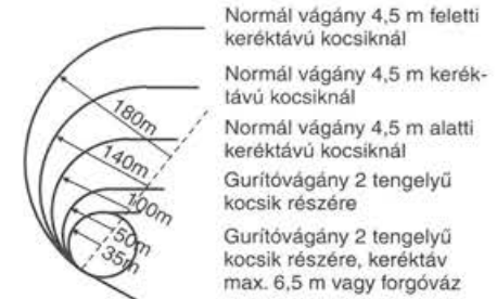
Kanyarodó vágány vágánsugara (forduló-képessége). Új vasutak építéseihez kerülni kell a 100 m-nél kisebb sugarakat.
