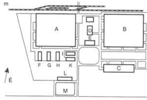
1.31. ábra. Alföldi Porcelángyár (tervező: Iparterv).
