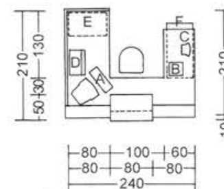
4.5. ábra. Ügyintéző-kifizető és tárgyalópultos munkahely méretei és berendezése.
