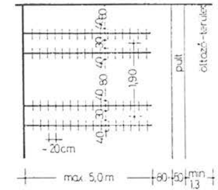
7.13. ábra. Fogasos elrendezés.
