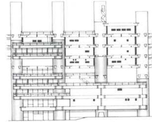
17.25. ábra. Kenzo Tange: Sajtó- és rádióközpont – Kofu, 1966.
