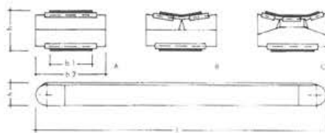
1.60. ábra. Szállítószalag.
