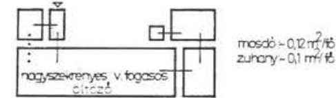
7.7. ábra. B típusú öltöző funkcióisméjája.
