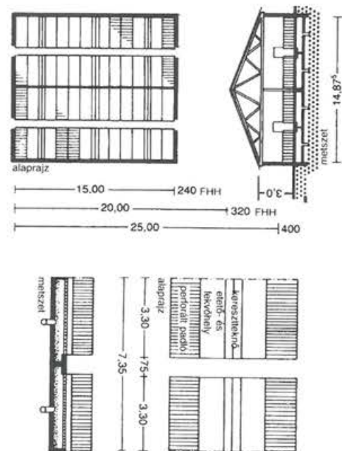
2.40. ábra. Kétszer kétsoros hizóistálló alaprajza, metszete.
