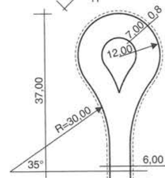
1.46. ábra. Gépkocsifordulók.
