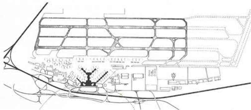
5.21. ábra. Frankfurt am Main légikikötőjének helyszínrajza.
