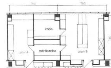
6.38. ábra. Berlin, Freie Universität laboratóriuma.
