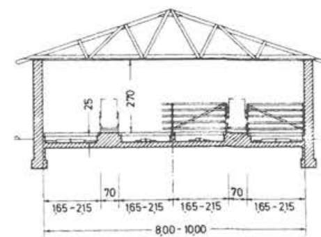
2.42. ábra. Vázás szerkezetű juhhodály alaprajza, metszete.
