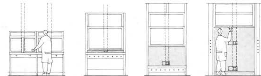
6.30. ábra. Helyi elszívók és vegyi fülkék
