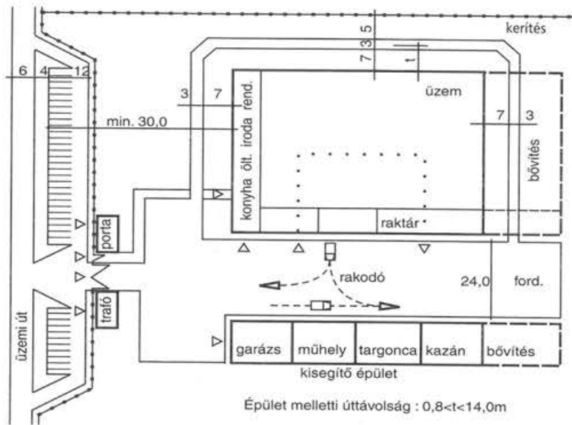
1.32. ábra. Üzemi épület általános elrendezése.
