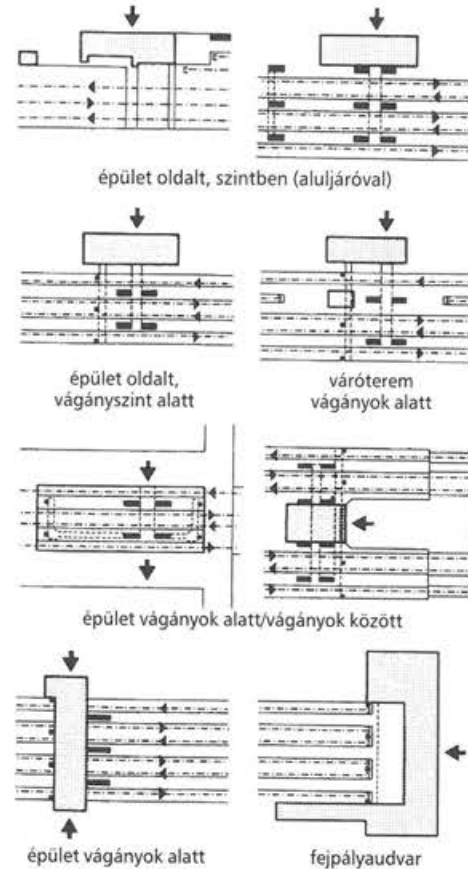
5.4. ábra. Fogadóépület-elrendezési sémák.
