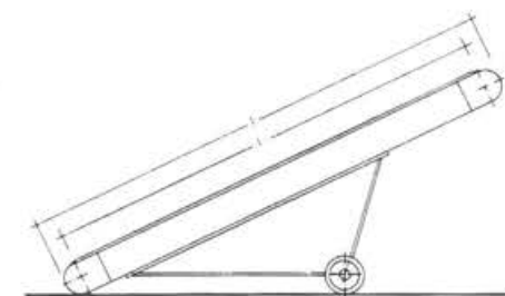
1.61. ábra. Szállítószalag.
