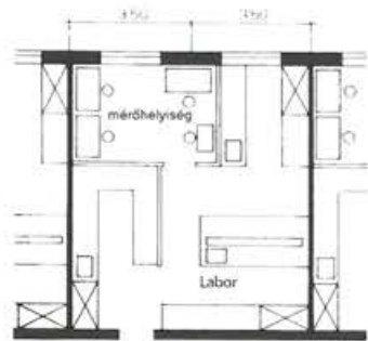
6.41. ábra. Laboratóriumok mérőhelyiséggel.
