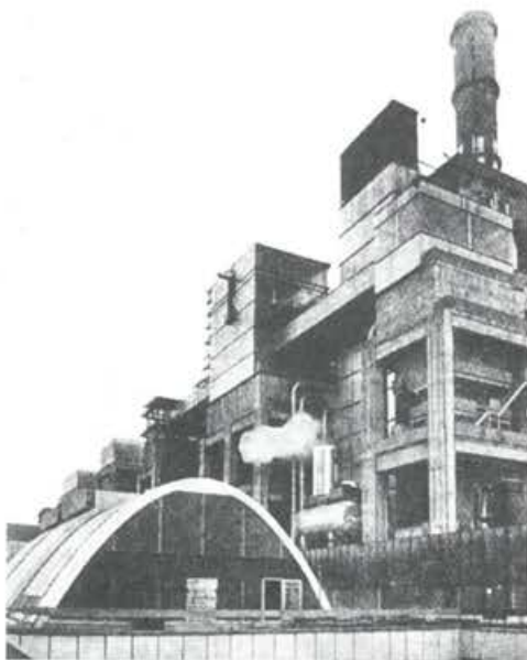
1.39. ábra. Erőmű félszabadtéri megjelenése. Mátrai Hőerőmű (építész-tervező: Springer Antal, Iparterv).
