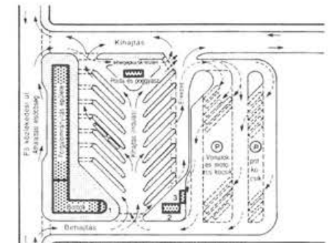
Nagy átmenő forgalmú pályaudvar a hozzá csatlakozó parkolóval
