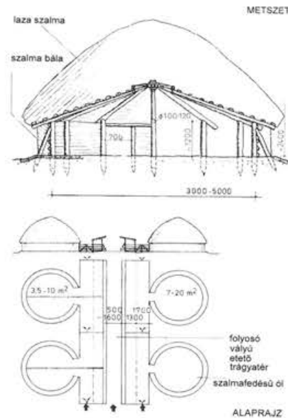
2.25. ábra. Kis költséggel előállított hízóól fedett etetővályúval.
