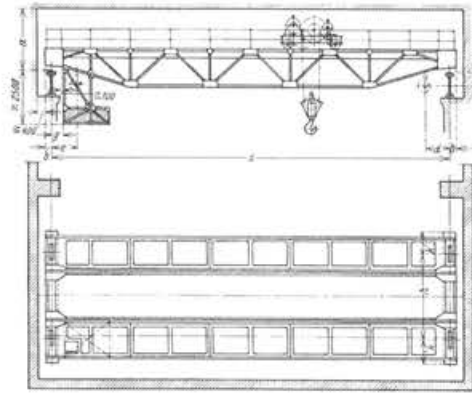
1.54. ábra. Híddaru, alaprajz-nézet.
