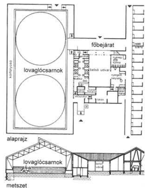
2.37. ábra. Lovarda (Gerolstein/Eifel), építész: Schnitzer.
