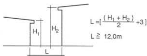
1.25. ábra. Épülettávolság.
