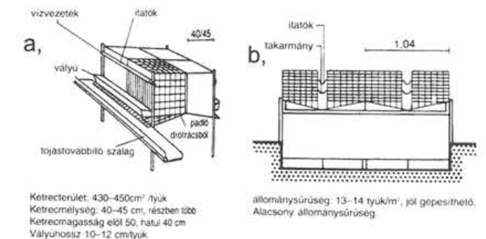
2.44. ábra. Ketreces tartás 1600 állat számára, istállóalaprész.
