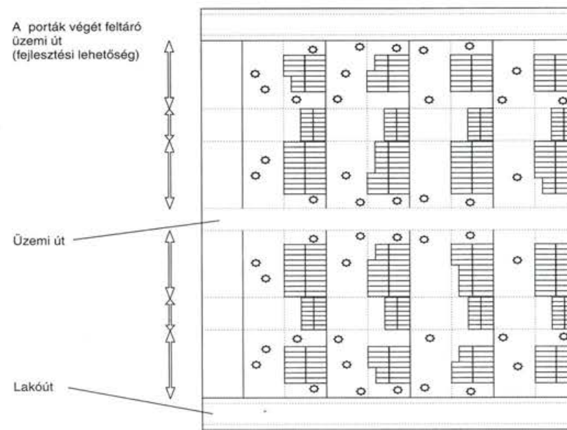
2.3. ábra. Üzemi út a porták között.
