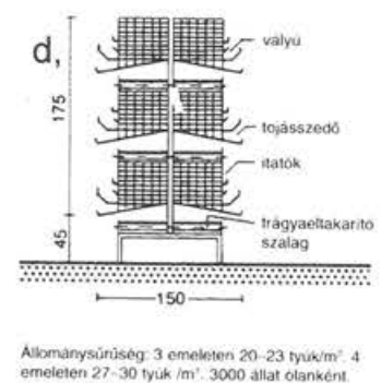
2.45. ábra. Ketrecek elrendezési változatai.
