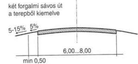
1.42. ábra. Egy és két forgalmi sávos közút mérete.
