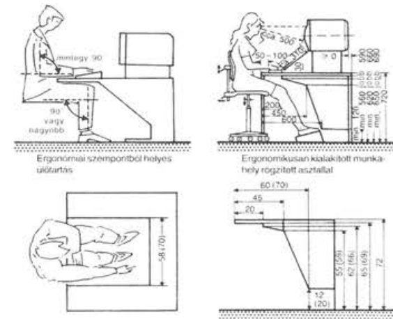
3.42. ábra. Irodai munkahely bútorzatának méretezése.
